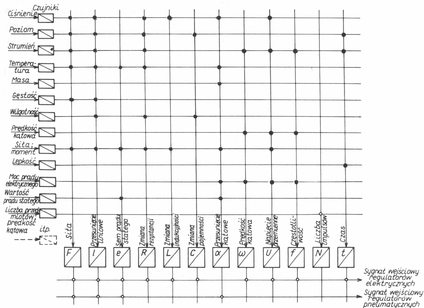
Rys. 3.2. Ideogram przetwarzania najczęściej mierzonych wielkości fizycznych (prof. dr hab. W. Findeisen — Technika automatycznej regulacji)
